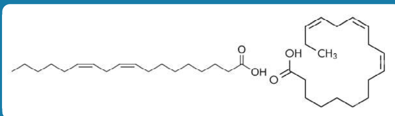
Figura 3. Estructura química del ácido linoleico (izq) y ácido \alpha -linolénico (der)(Med Chem Express, s.f & Alamy, 2021).
