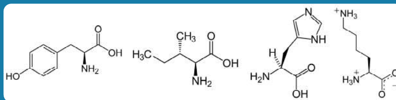
Figura 2. Estructura química de la tirosina, isoleucina, histidina y lisina (de izq a der) (Benjah, 2006 & Neurotiker, 2007 & Mills, 2009).
